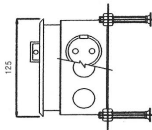
SYSTEM BOX 측면도
