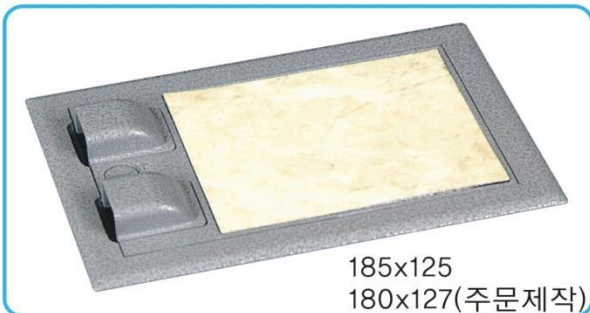
AL 커버
