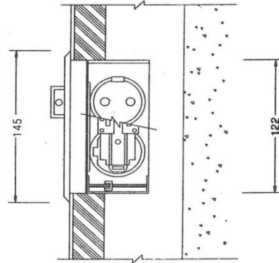
SYSTEM BOX 평면도
