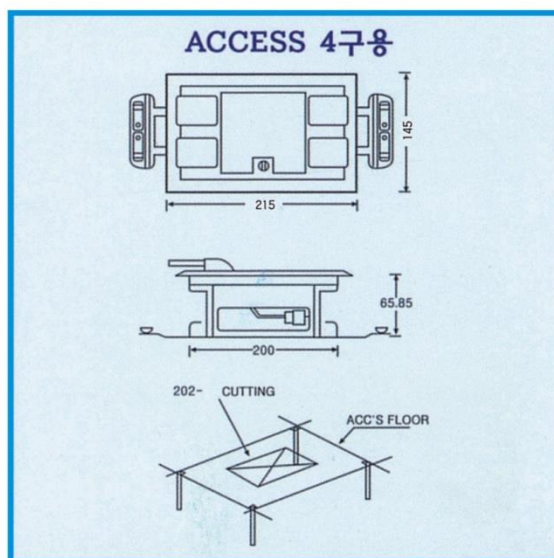
부품 조립도
